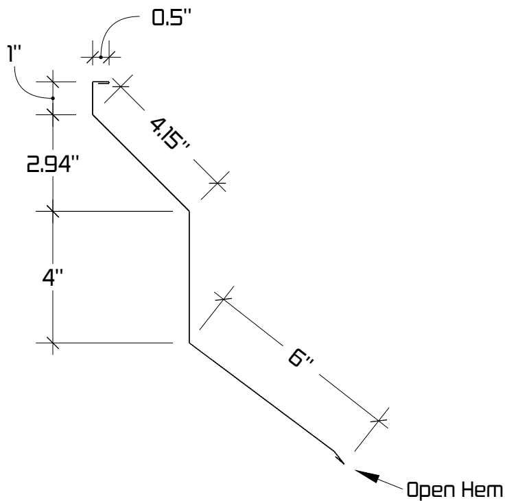
Bottom Apron Louver Blade
