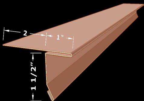
Locking Edge Metal
